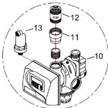
DETALLE
