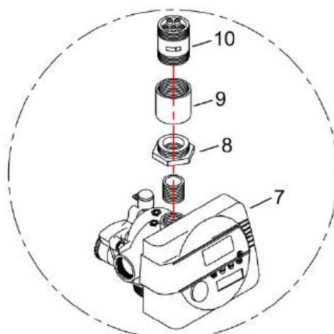
DETALLE
