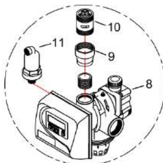
DETALLE
